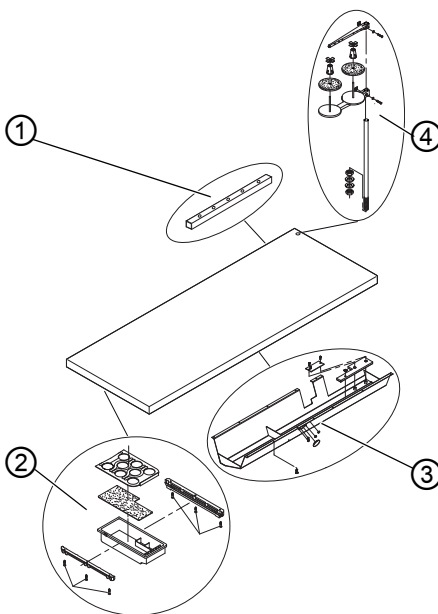
Image 53: Compléter la table
