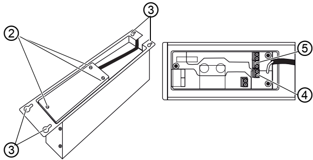
Image 61: Raccorder le transformateur de lampe de couture (2)
