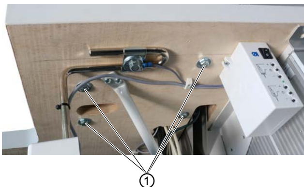
Image 57: Installer la tête de machine (1)
