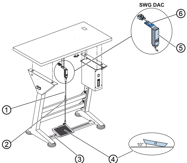
Image 52: Montage de la pédale du dispositif de valeur de consigne
