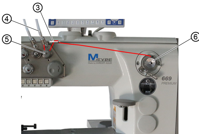
Image 10: Bobiner le fil de crochet (2)
