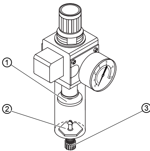
Image 50: Nettoyer l'élément filtrant
