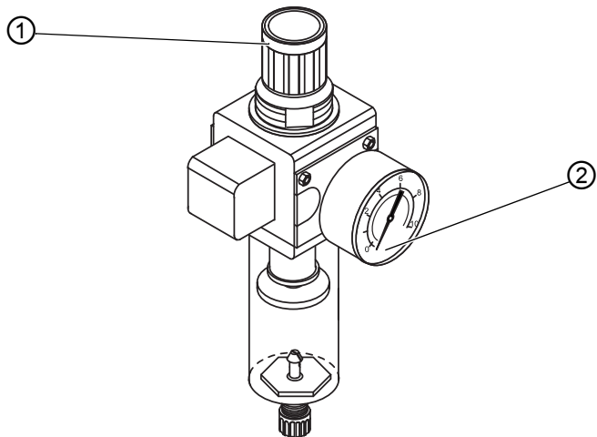
Image 48: Régler la pression de service
