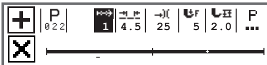
Image 38: Affichage en mode de programmation
