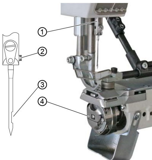
Image 4: Mettre en place ou changer l'aiguille
