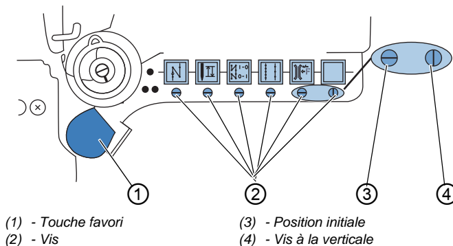
Image 21: Affecter une fonction à la touche favori
