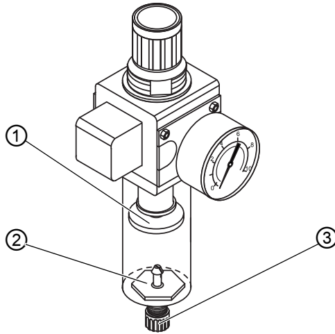
Image 49: Évacuer l'eau de condensation
