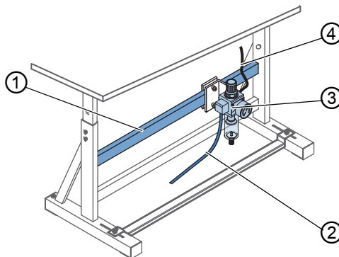
Image 63: Monter l'unité de maintenance à air comprimé
