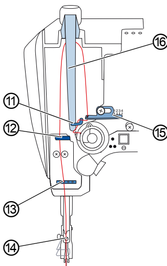
Image 7: Enfiler le fil d'aiguille (3)
