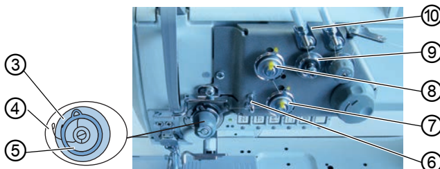
Image 6: Enfiler le fil d'aiguille (2)
