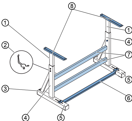
Image 51: Montage du bâti
