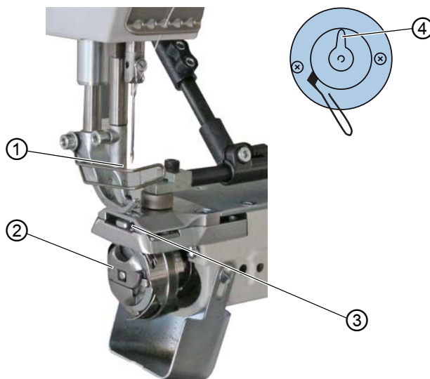
Image 45: Endroits dont le nettoyyage est particulièrement important
