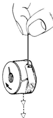
Image 14: Régler la tension du fil de crochet (1)
