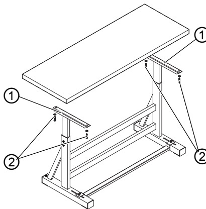
Image 54: Fixation de la table au bâti
