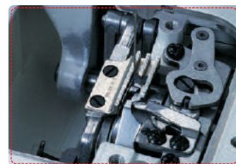
● Coupe-Fil Automatique Avec votre coupe-fil automatique, vous pouvez couper à la fois le fil de l'aiguille et le fil de la canette simultanément. Profitez de la technologie de l'inventeur du coupe-fil ! Sur cette machine, il s'agit du même mécanisme que nos machines à coudre JUKI industrielles.
