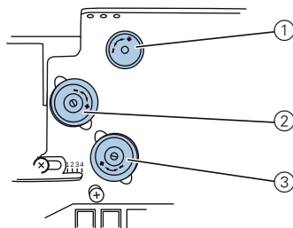
Fig. 17: Régler la tension du fil d'aiguille
