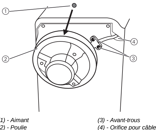
Fig. 67: Monter le capteur à effet Hall
