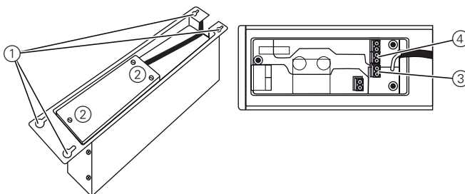
Fig. 63: Brancher le transformateur de la lampe de couture à l'unité de contrôle DAC
