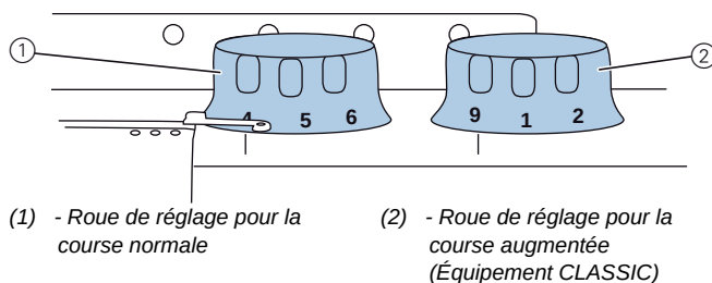
Fig. 28: Roue de réglage pour la course des pieds presseurs
