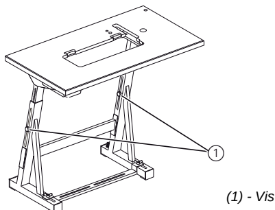
Fig. 52: Régler la hauteur de la table de travail
