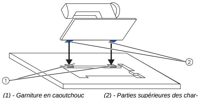
Fig. 55: Mettre la tête de machine en place
