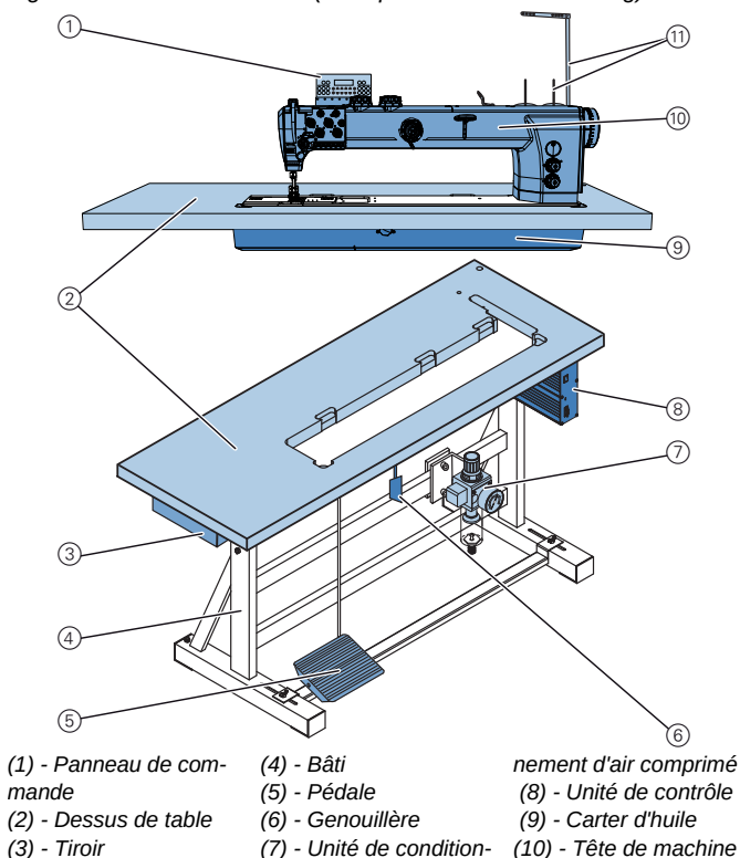
Fig. 47: Étendue de livraison (exemple: Machine à bras long)
