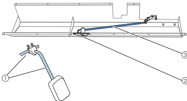
Fig. 57: Monter la genouillère mécanique
