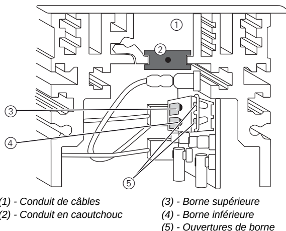
Fig. 64: Brancher le transformateur de la lampe de couture à l'unité de contrôle Efka
