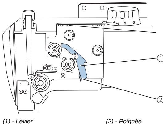
Fig. 19: Activer et désactiver la tension supplémentaire - machines ECO
