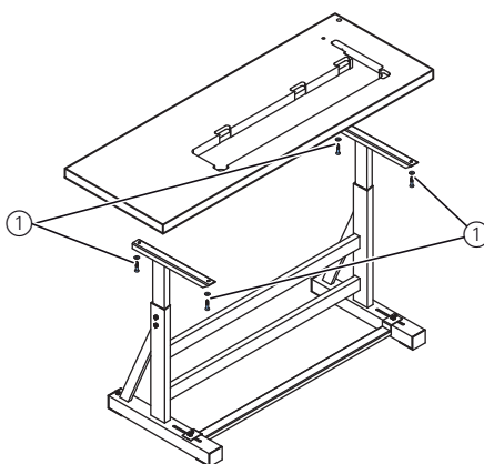
Fig. 51: Fixer le dessus de table sur le bâti
