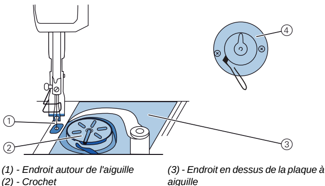
Fig. 41: Endroits nécessitant un nettoyage particulier
