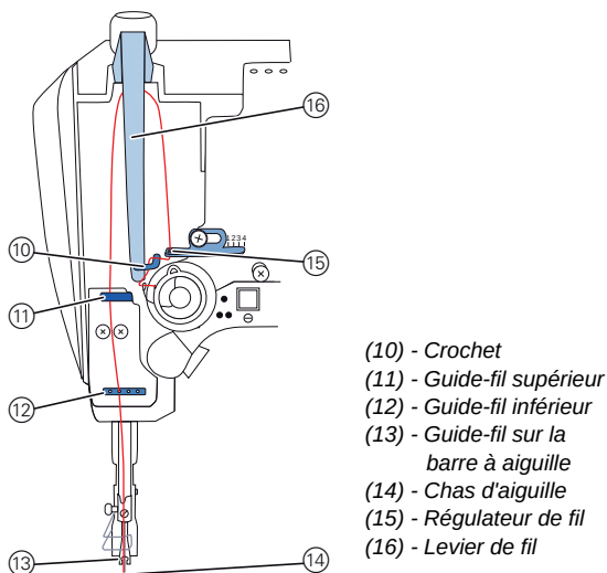
Fig. 8: Schéma d'enfilage - partie 2
