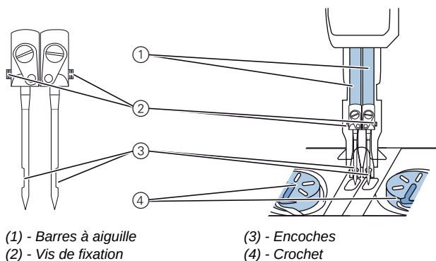
Fig. 5: Insérer et changer d'aiguille sur les machines à barres à aiguille commutables
