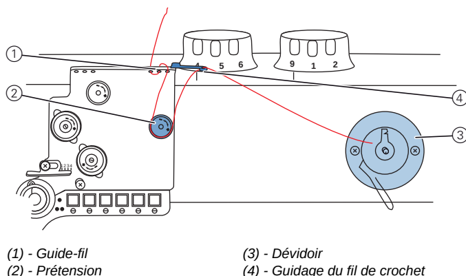
Fig. 12: Bobiner le fil de crochet - partie 1
