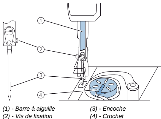
Fig. 3: Insérer et changer d'aiguille sur les machines à aiguille
