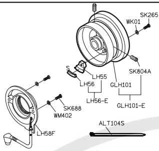
旋轉式切刀
