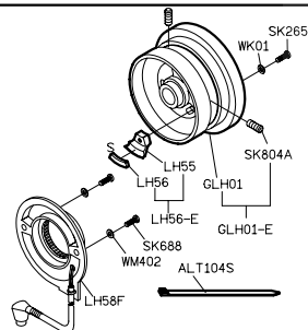
擺動式切刀
