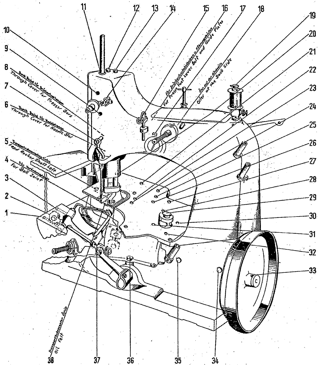
ÖL-DIAGRAMM LUBRICATING DIAGRAM
