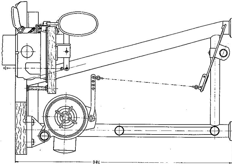
Schnitt A-B
