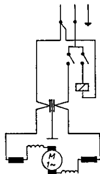
WIRING-DIAGRAM SCHALTPLAN
