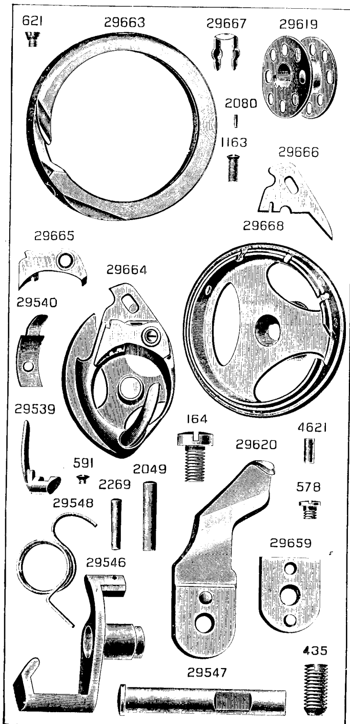
PLATE 3506—FULL SIZE
