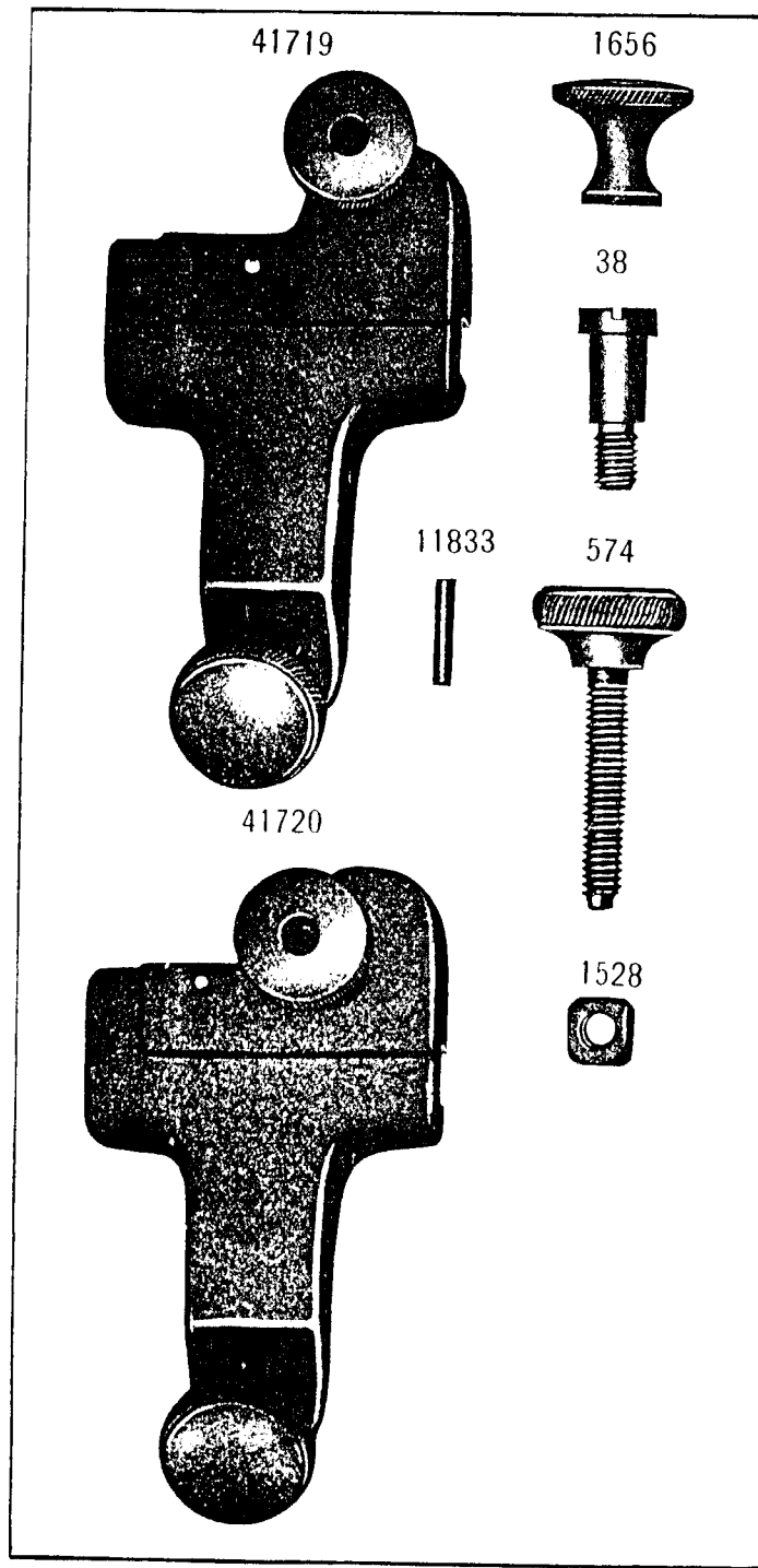
PLATE 6536—FULL SIZE
