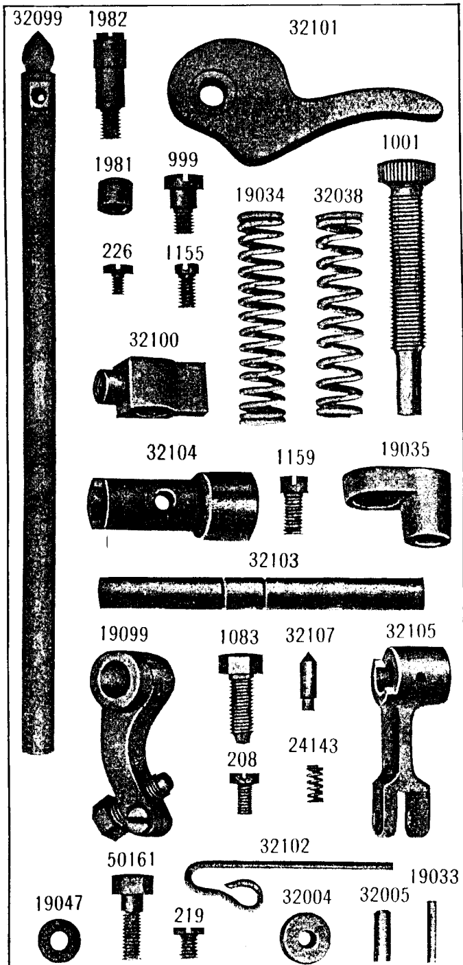
PLATE 2194—FULL SIZE
