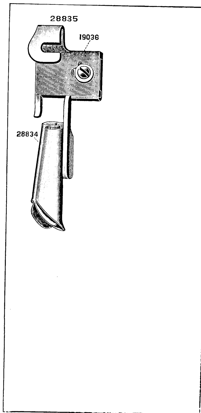
PLATE 2172—FULL SIZE
