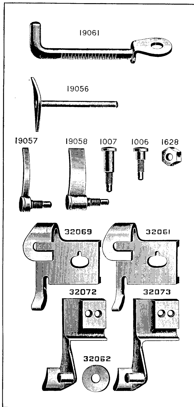
PLATE 2157—FULL SIZE
