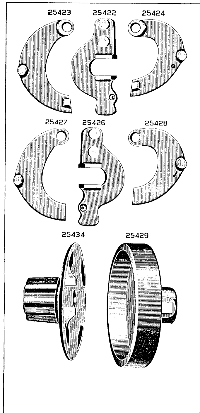
PLATE 3815—ONE-HALF SIZE
