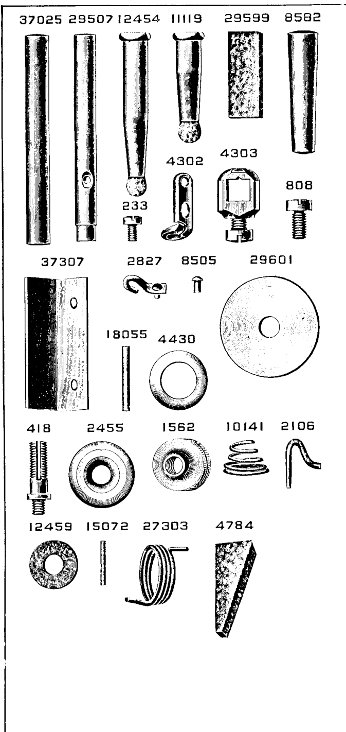
PLATE 6114—FULL SIZE
