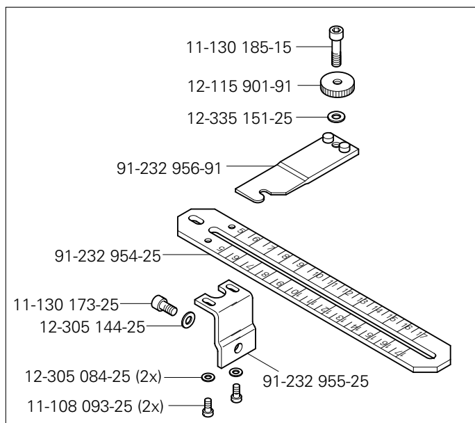
91-232 953-90 (PFAFF 3307 -1/01; -1/02)
