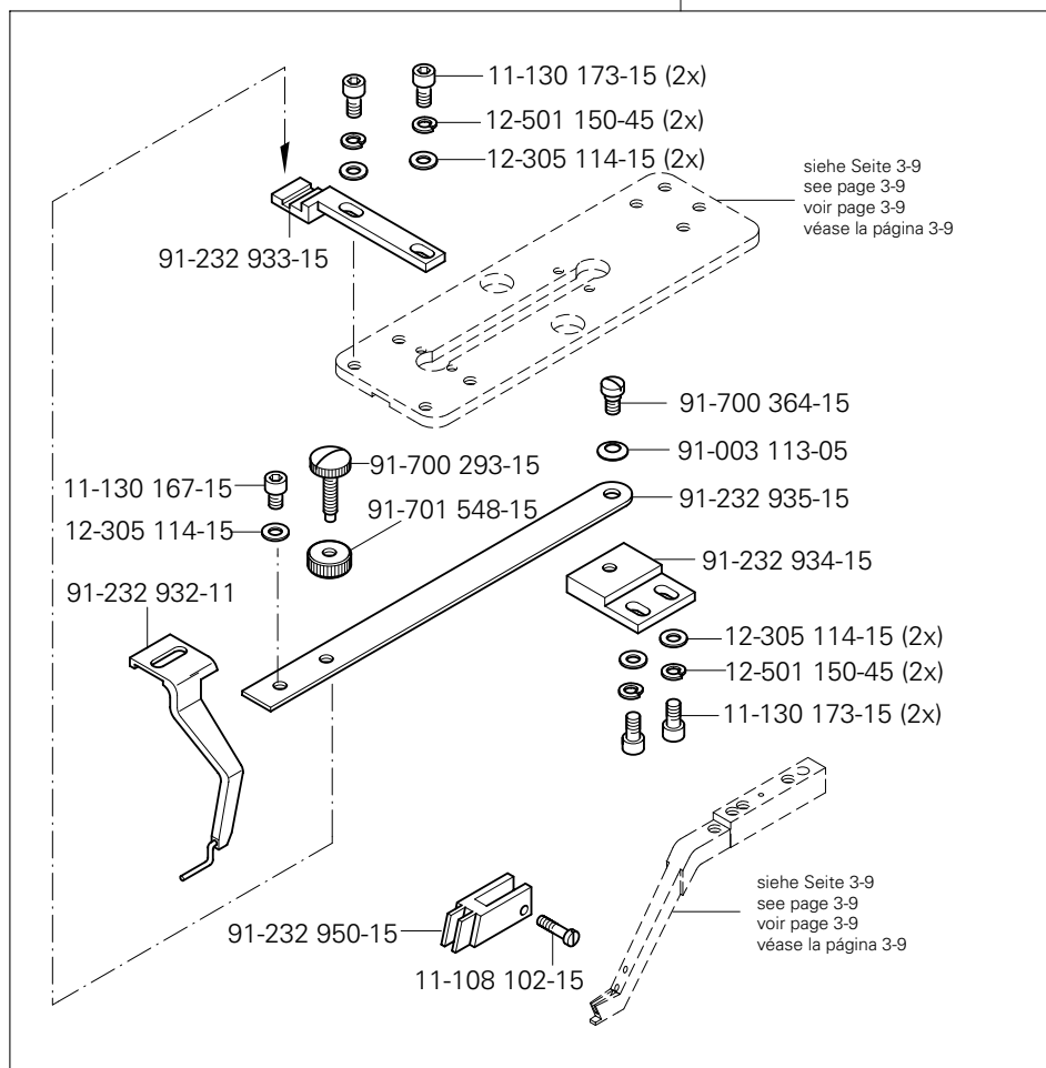
91-232 952-90 (PFAFF 3307 -1/01; -1/02; -1/03; -5/01)
