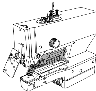
91-232 952-90 (PFAFF 3307 -1/01; -1/02; -1/03; -5/01)
